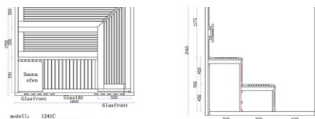
modell: 1241C Abmessungen: 1800*1700*600 Einheit: MM
