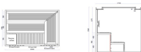
modell: 1241B Abmessungen: 2000*1700*600 Einheit: MM
